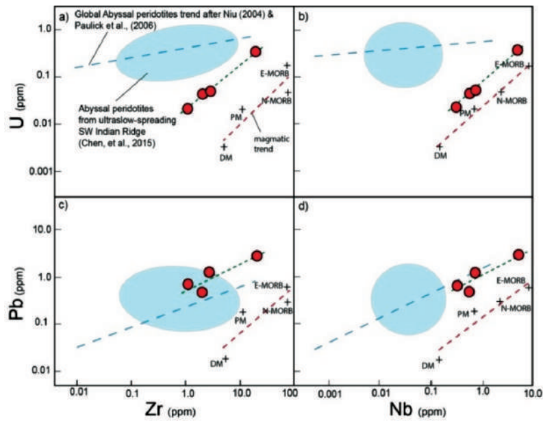
شکل ۹. a-d) نمودارهای عناصر زیرکونیوم و نئوبیم در برابر اورانیم و سرب برای سرپانتینیت‌های غرب ماکو که در آن روند تحولات ماگمایی و نیز موقعیت گوشته تهی شده، غنی شده و بازالت‌های پشته میان اقیانوسی عادی و غنی شده مشخص شده‌اند، بعلاوه پریدوتیت‌های اقیانوسی‌های با گسترش کند با رنگ آبی مشخص شده و مرجع داخل شکل آمده است
