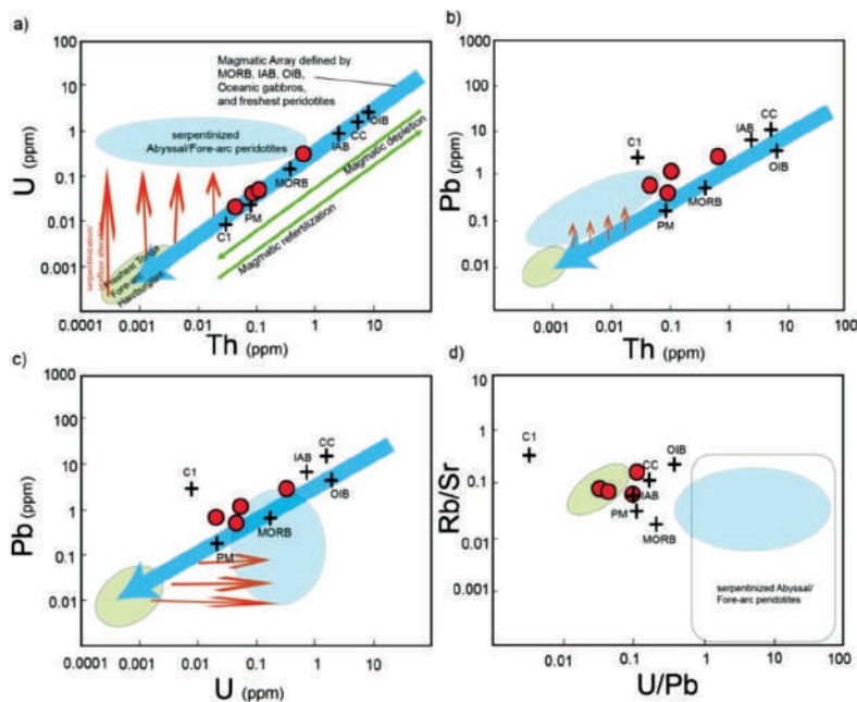
شکل ۱۰. a-d) نمودارهای تعیین محیط تکتونیکی برای سرپانتینیت‌های غرب ماکو، بعلاوه موقعیت پریدوتیت‌های مناطق عمیق، بازالت پشته میان اقیانوسی، بازالت جزایر قوسی، گابروی اقیانوسی، پریدوتیت‌های جلوی قوسی گودال ماریانا و نیز پریدوتیت‌های جلوی قوسی تونگا مشخص شده است، MORB, Niu et al. (1999); IAB, Ewart et al. (1998) from Mariana and Tonga; oceanic gabbros, Bach et al. (2009), Niu et al. (2002), Niu and O'Hara (2003). Average OIB, PM and C1 values are from Sun and McDonough (1989) .. and CC (bulk continental crust) from Rudnick and Fountain (1995)
